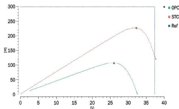
Curva caratteristica POT / OPC+STC
