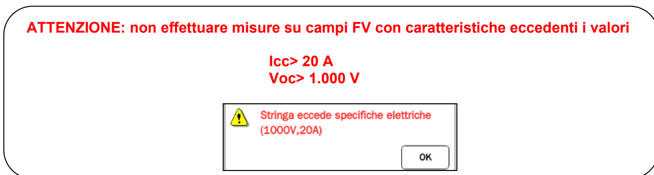
Figura 14.7.3-10 c Schermata di errore: valori di corrente e tensione che eccedono i valori massimi in ingresso
