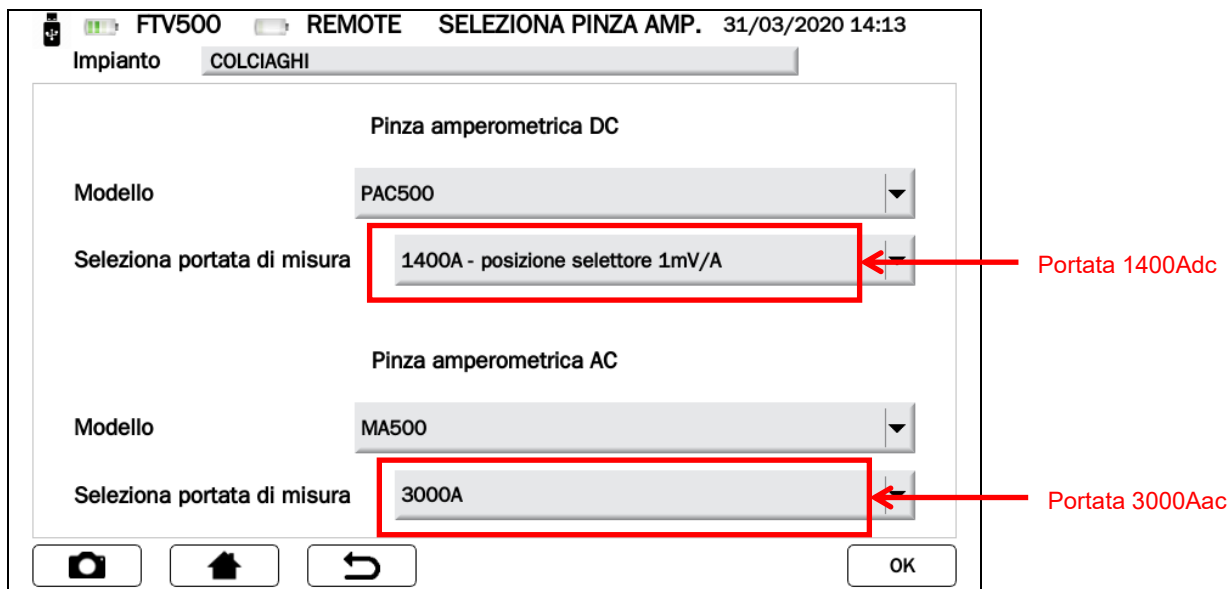
Figura 14.7.2-5 Schermata Seleziona Pinza Amperometrica
