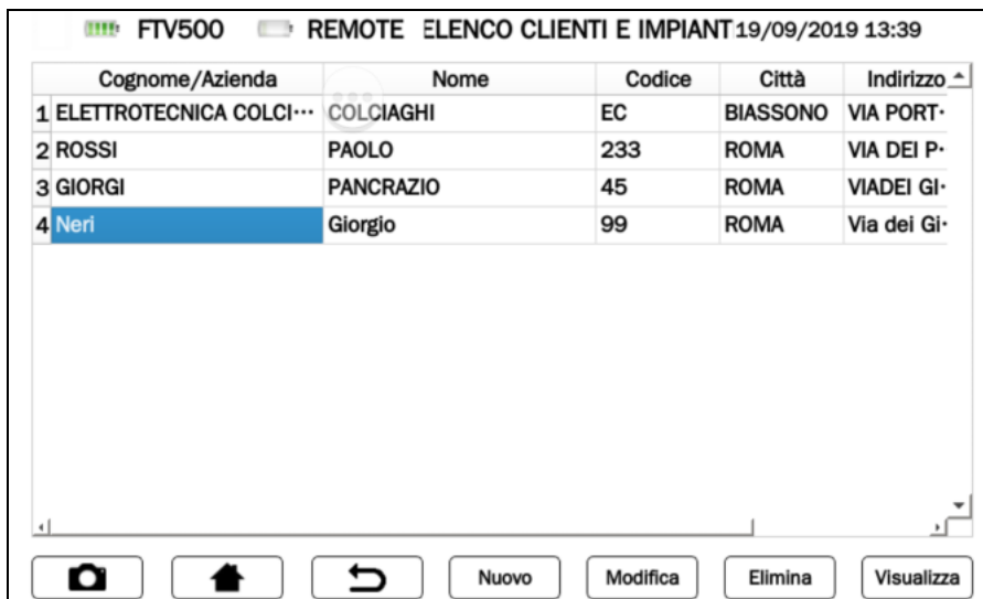
Figura 14.3.2-4 Schermata lista clienti per NUOVO IMPIANTO
