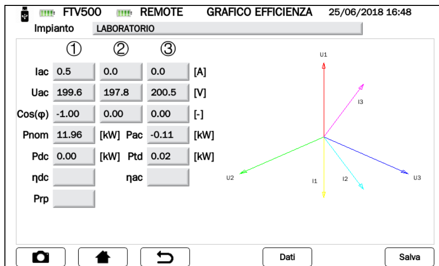
Figura 14.7.1-11 Schermata Visualizzazione Grafico Efficienza
